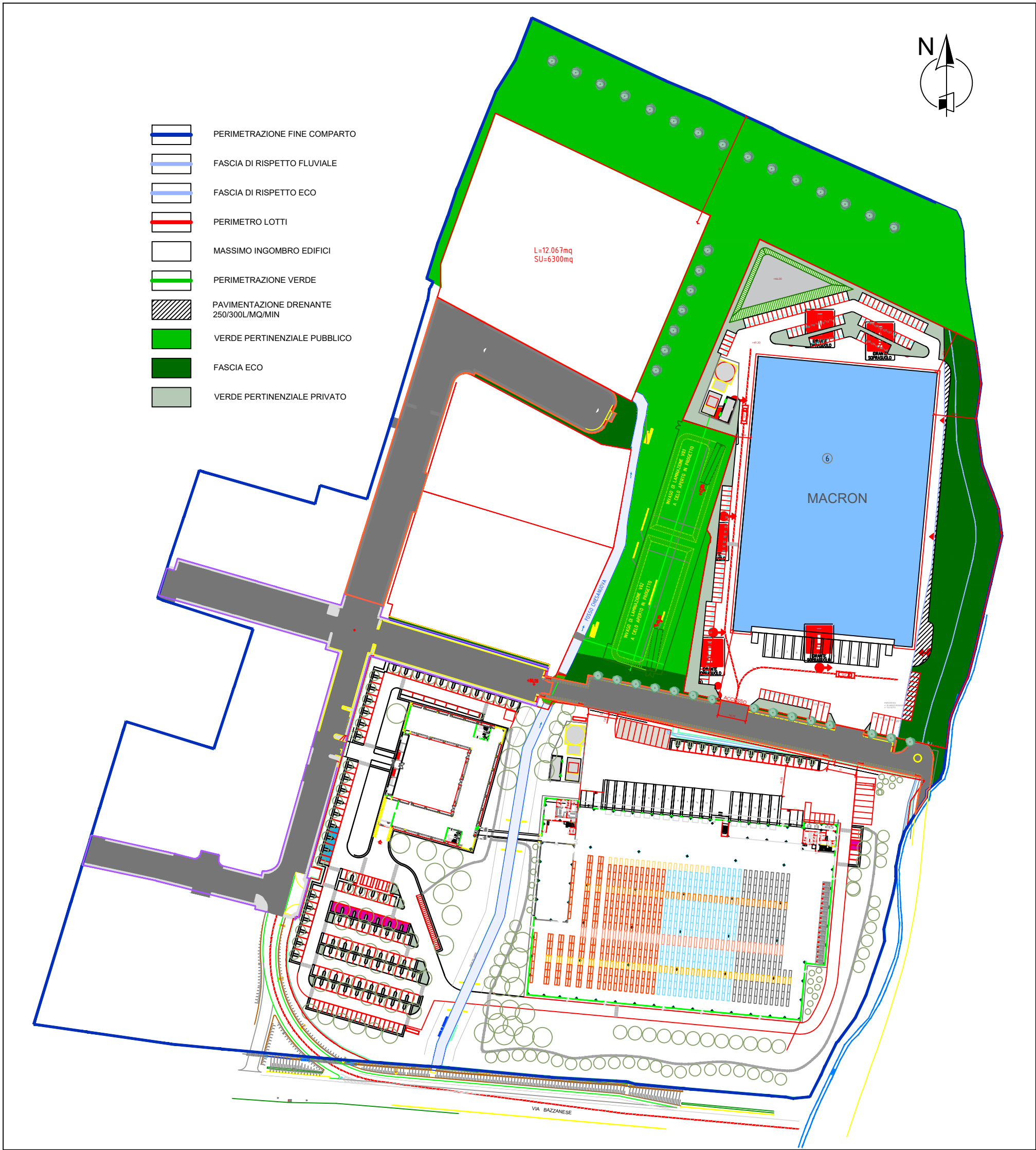
Planimetria Generale - Scala 1:2000
